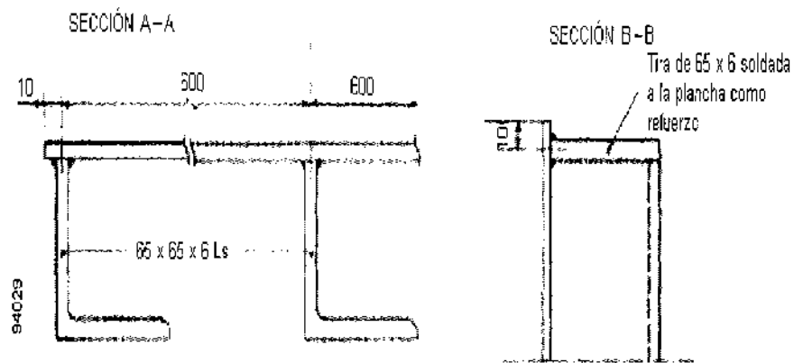
Figura 1 – Núcleo estructural de acero para mamparos de clase "A" y revestimientos de clase "B"
