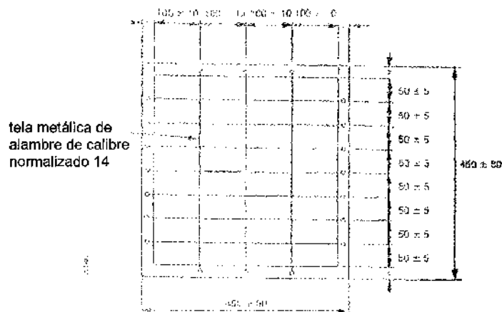
b) Espaciamento de la plataforma de tela metálica
