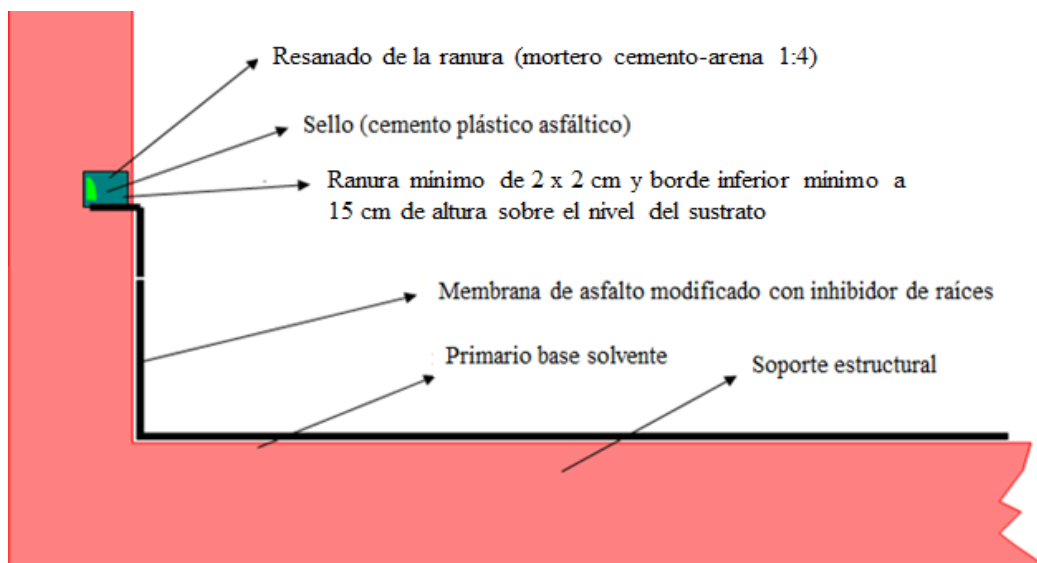
Figura 10. Esquema de fijación de membrana asfáltica a pretils, muretes y similares.
