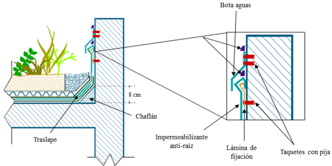
Figura 7. Impermeabilización con láminas de PVC, propileno-etileno o similares en puntos de encuentro con pretiles y elementos emergentes perimetrales.
