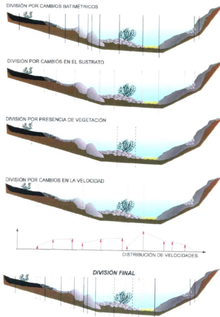
Figura E.4. Ubicación de los puntos a tomar en aquellas singularidades del lecho; se modifica la anchura de las celdas con el fin de obtener mayor precisión en la determinación de su perfil.
