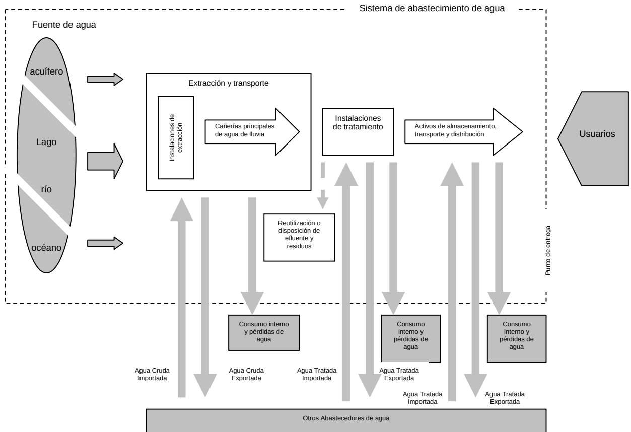
Figura A.2 — Esquema de un servicio de abastecimiento de agua potable centralizado típico
