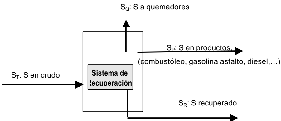
Figura 1. Balance de azufre de una refinería
