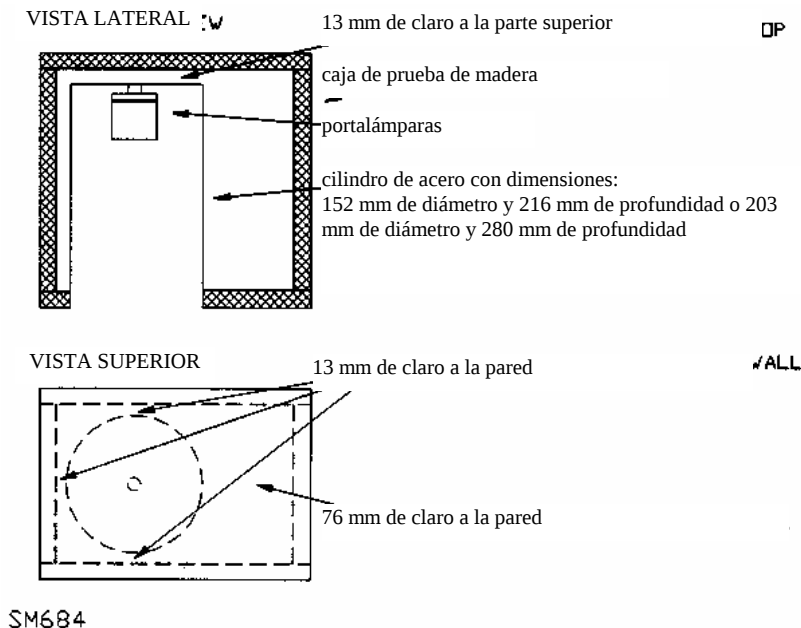
Figura 1.- Luminario de prueba
