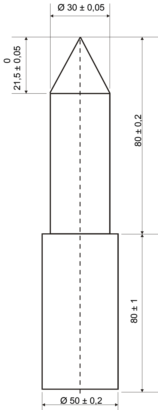
Figura 4. Probeta de prueba Dimensiones en mm
