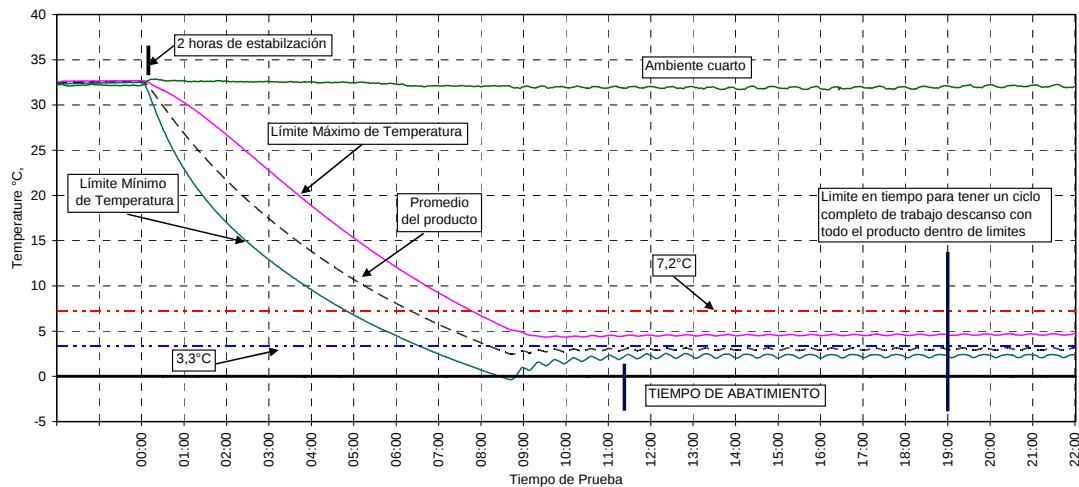
Gráfico Prueba de Abatimiento de Temperatura "pull down".
