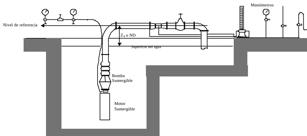
Figura 1.- Instalación típica para conjunto motor bomba sumergible.
