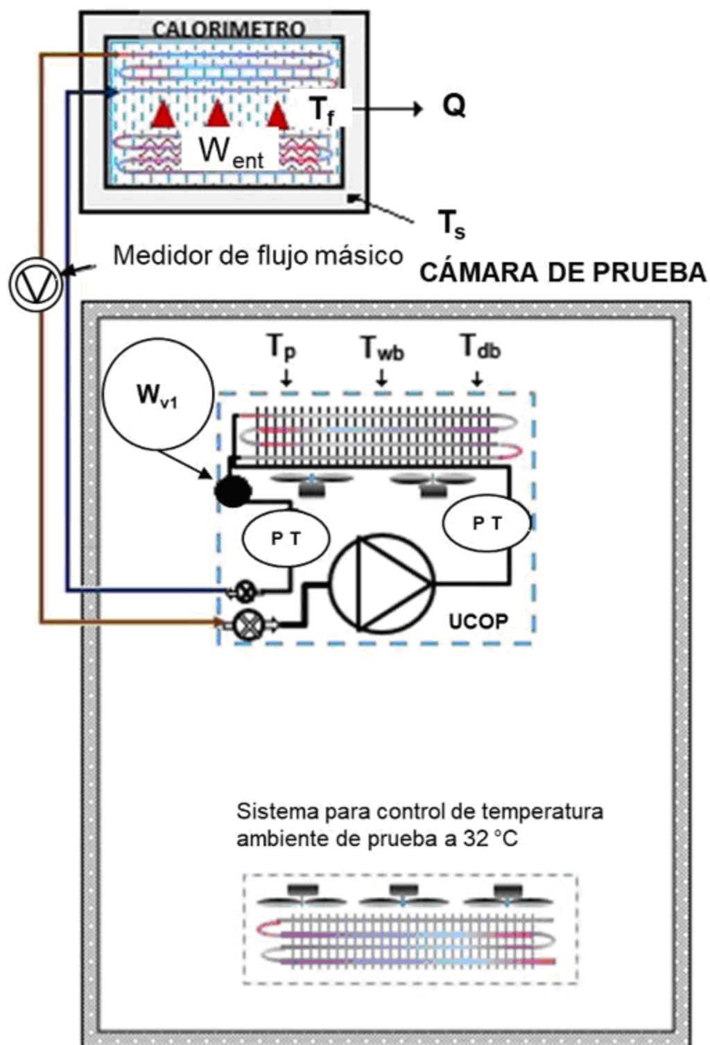
Figura 5 - Método calorímetro
