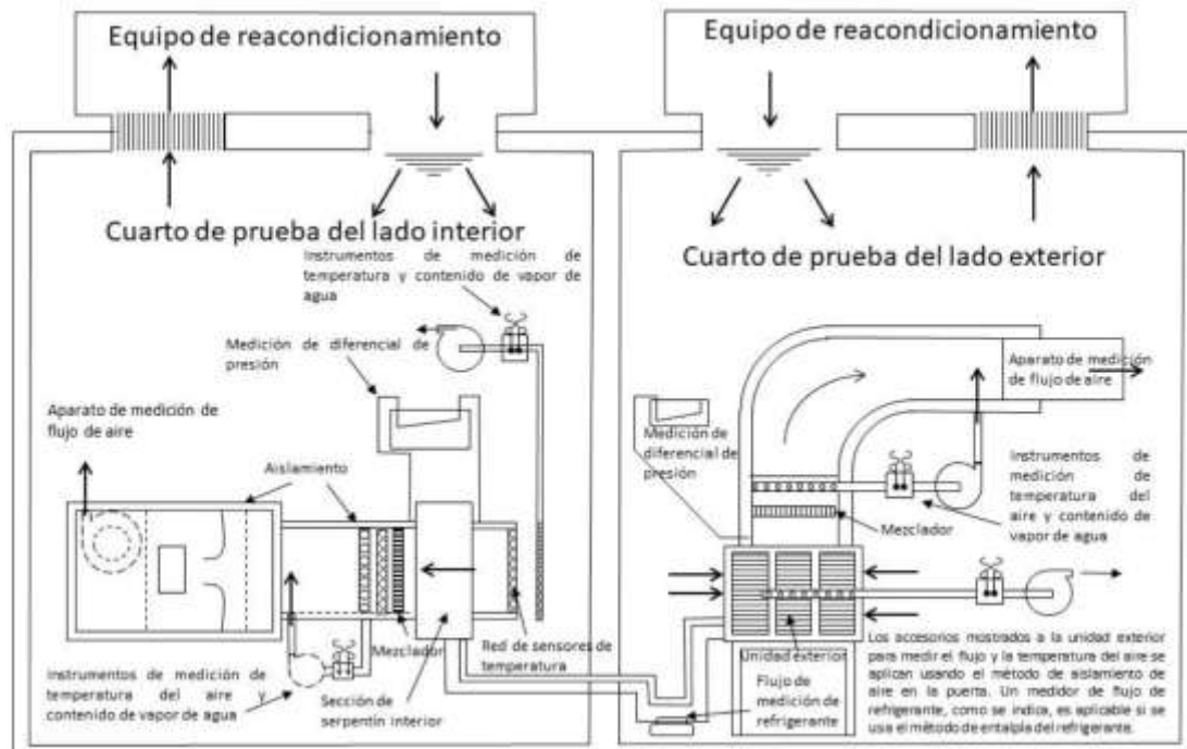
Figura A.1-Método de túnel aire-entalpía
