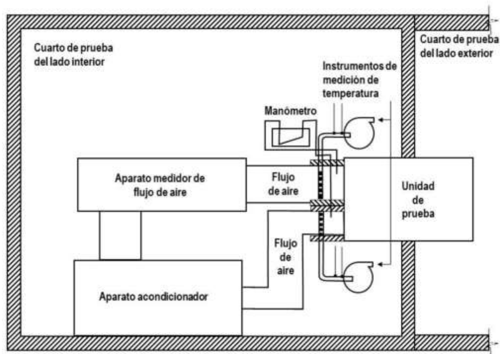
Figura A.2-Método de enlace de aire-entalpía
