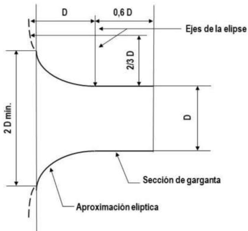
Figura A.6-Tobera para la medición del flujo de aire
