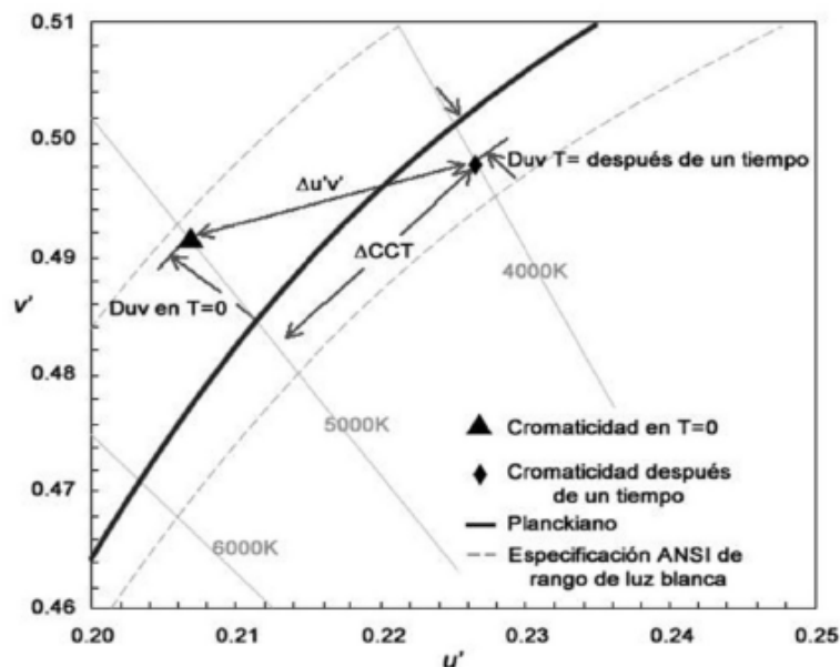
Figura L1 - Diagrama de cromaticidad que ilustra la diferencia entre \Delta u'v' , \Delta Duv y \Delta TCC
