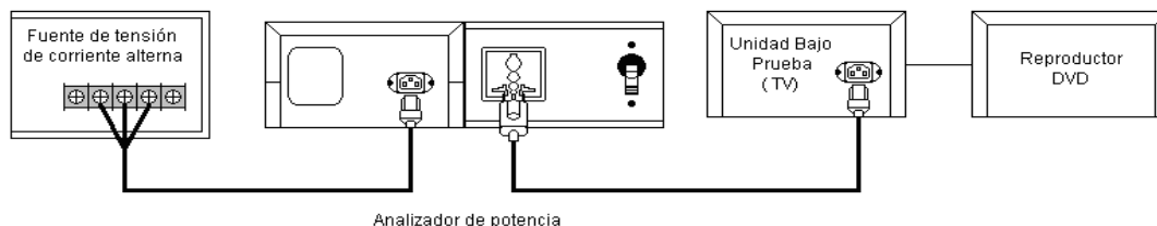
Figura 7. Arreglo de pruebas para las mediciones de potencia eléctrica en modo de espera.
