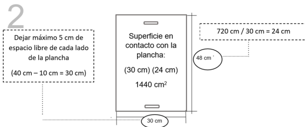
Figura E.6 – Ejemplo de las dimensiones de la superficie de la olla de BoPET para cada una de las dos ollas en contacto con la plancha de 40 cm por 60 cm
