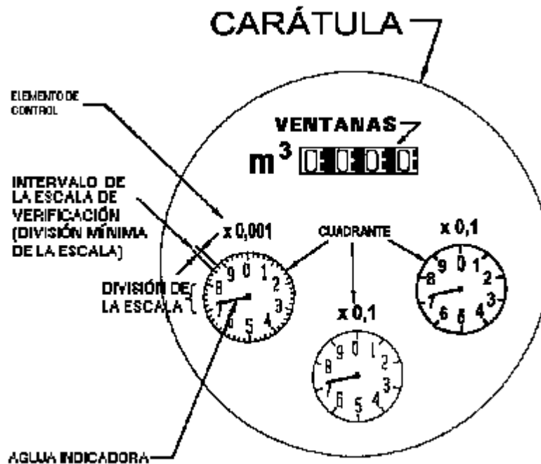
FIGURA 5A.- Tipo 3 Dispositivos analógicos y digitales combinados
