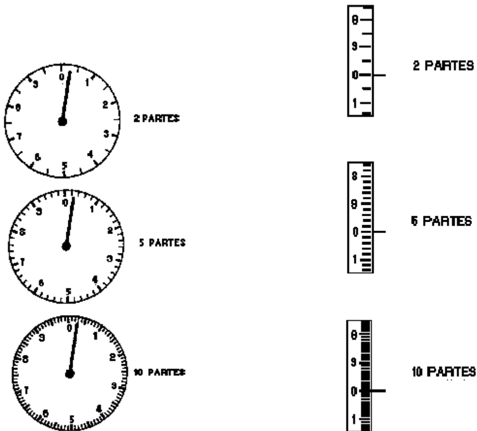
FIGURA 7A.- Valor de la división mínima de verificación
