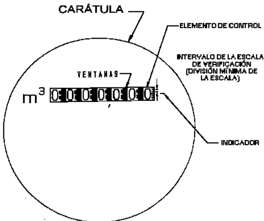
FIGURA 4.- Tipo 2 Dispositivo digital
