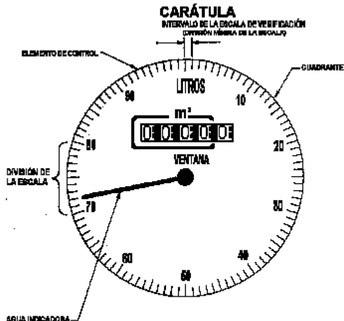
FIGURA 5B.- Tipo 3 Dispositivos analógicos y digitales combinados
