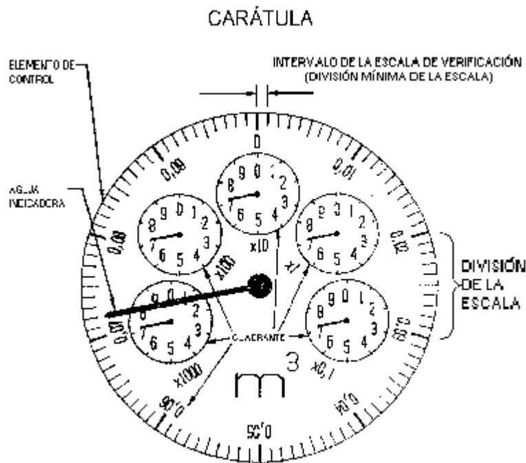
FIGURA 3.- Tipo 1 Dispositivo analógico
