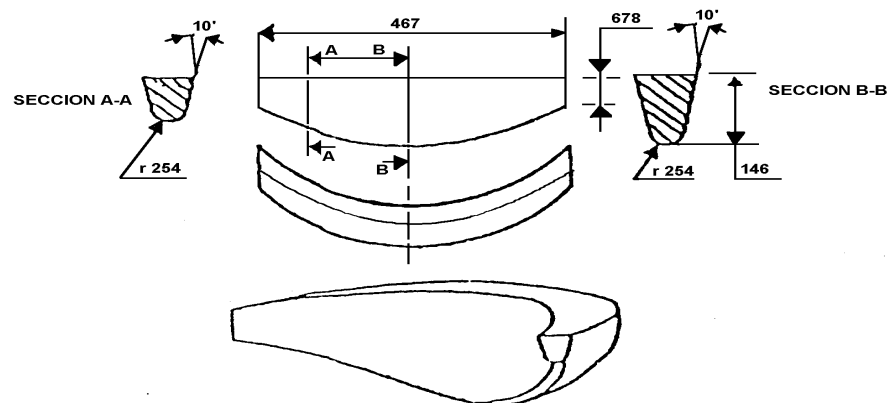
FIGURA 1.- Esquema de referencia de un equipo de prueba de resistencia de la ceja al desmontaje del rin.
