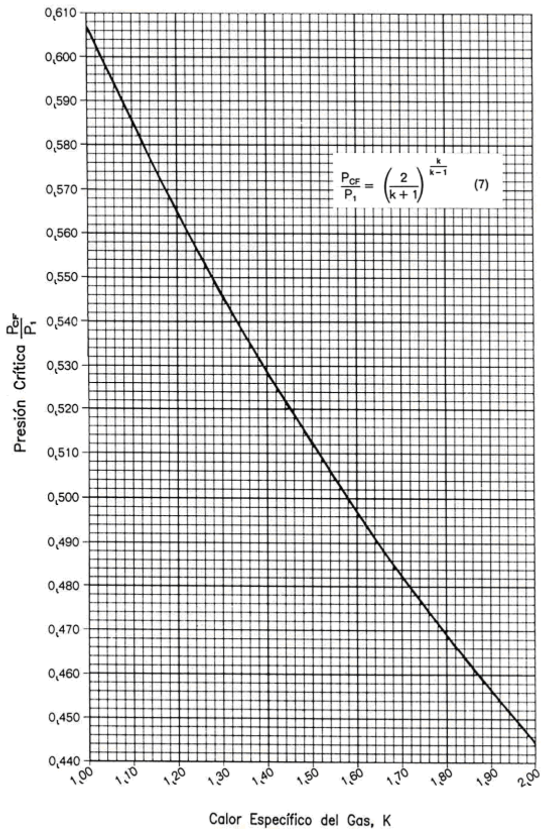
Figura ilustrativa C2 - Curva para determinar el valor de la presión crítica P_{ct}/P_1
