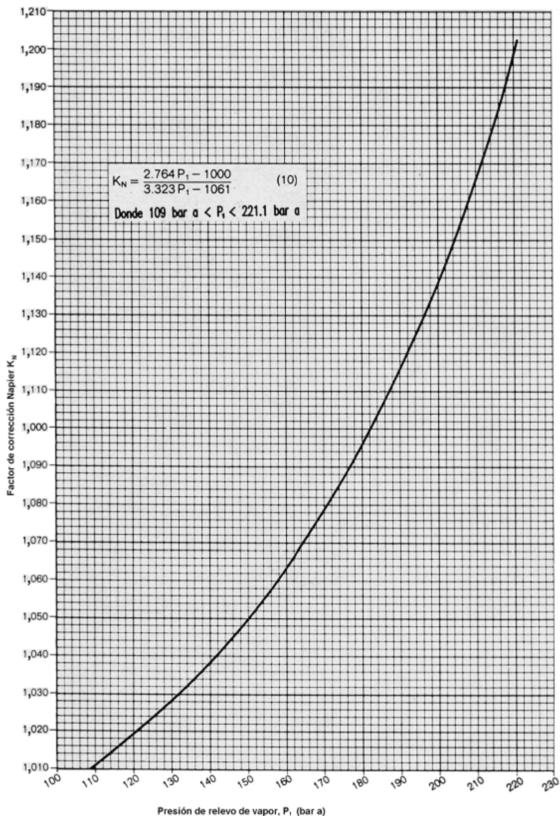
Figura ilustrativa C6 - Curva para determinar el factor de corrección K_N de Napier para altas presiones de vapor saturado seco.
