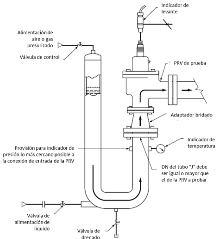
Figura ilustrativa 11 - Arreglo recomendado para banco de pruebas para fluidos incompresibles.
