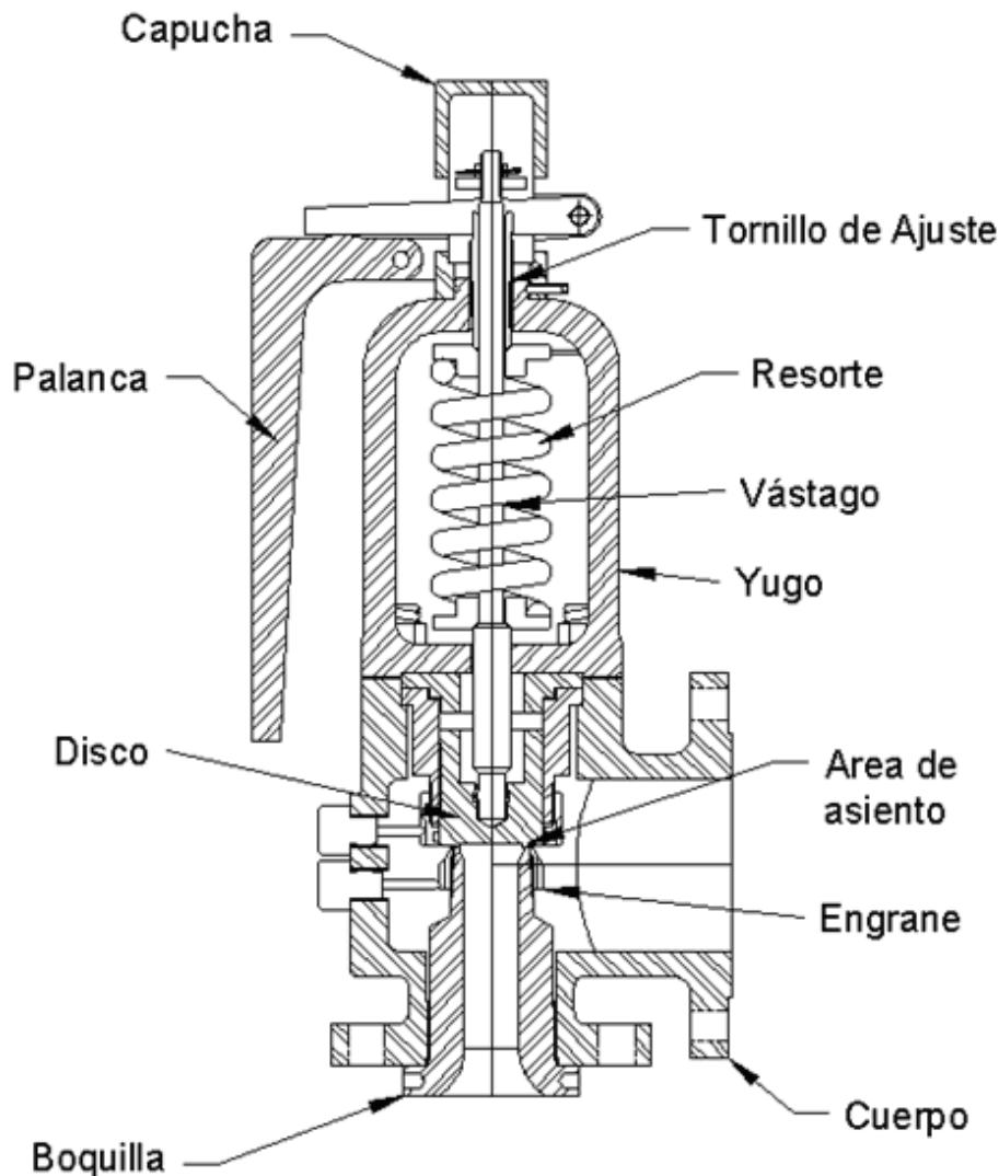
Figura 1.- Válvula de Seguridad
