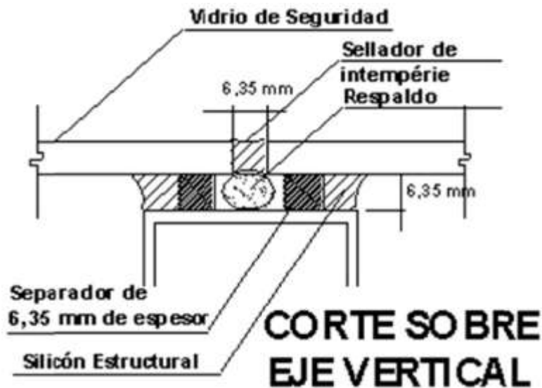
Figura 8.- Corte del envidriado sobre el eje vertical
