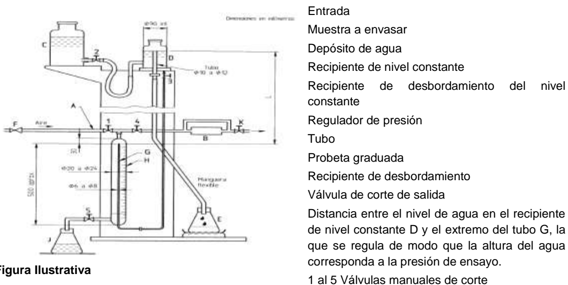
Figura A.1-Dispositivo para la verificación de la hermeticidad del circuito de gas (Método volumétrico) (Ver 7.11 y Apéndice A)
