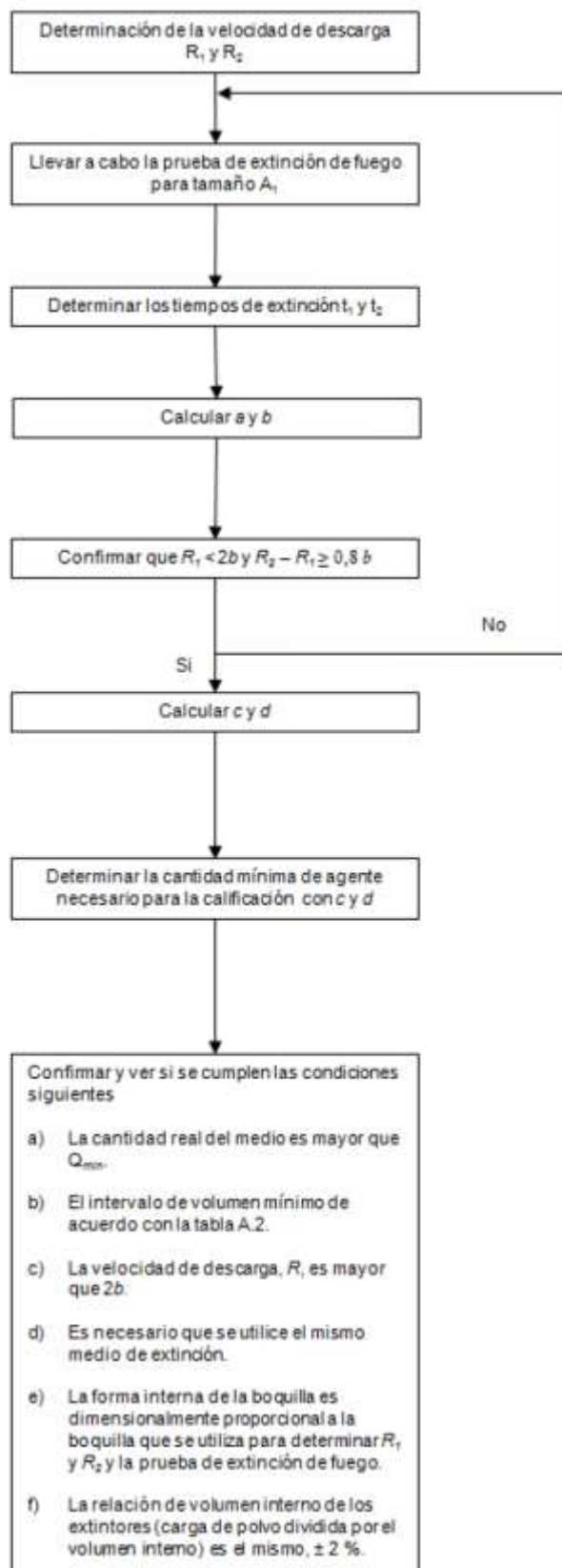
Figura A.1 Método de prueba alternativo de evaluación de un extintor con polvo como agente extinguidor que tiene una capacidad que superar 144B
