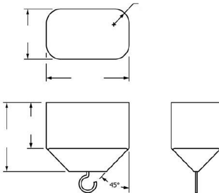
Figura 4-Bloque de cuña
