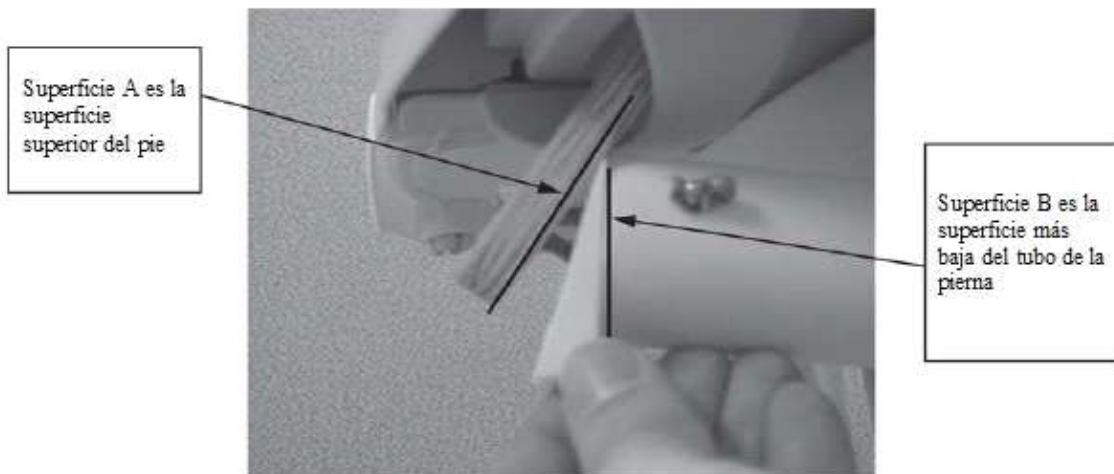
Figura 6-Bloque de 30°
