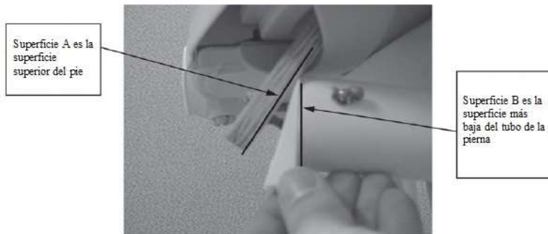
Figura 7 - Bloque de 30°
