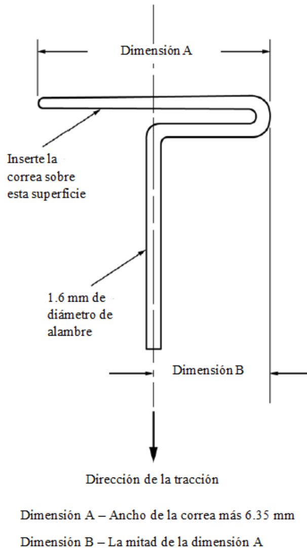
Figura 4 - Dispositivo de tracción
