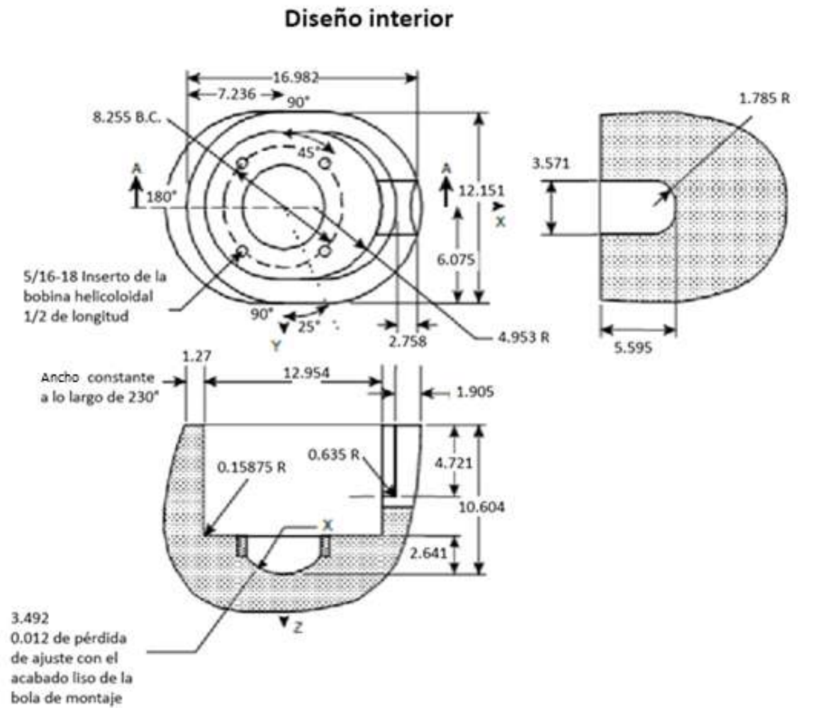
Figura A.3-Cabeza de referencia pequeña
