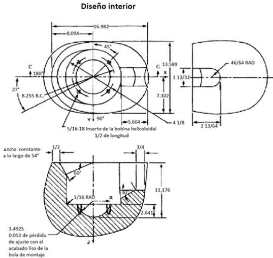
Figura A.4-Cabeza de referencia mediana
