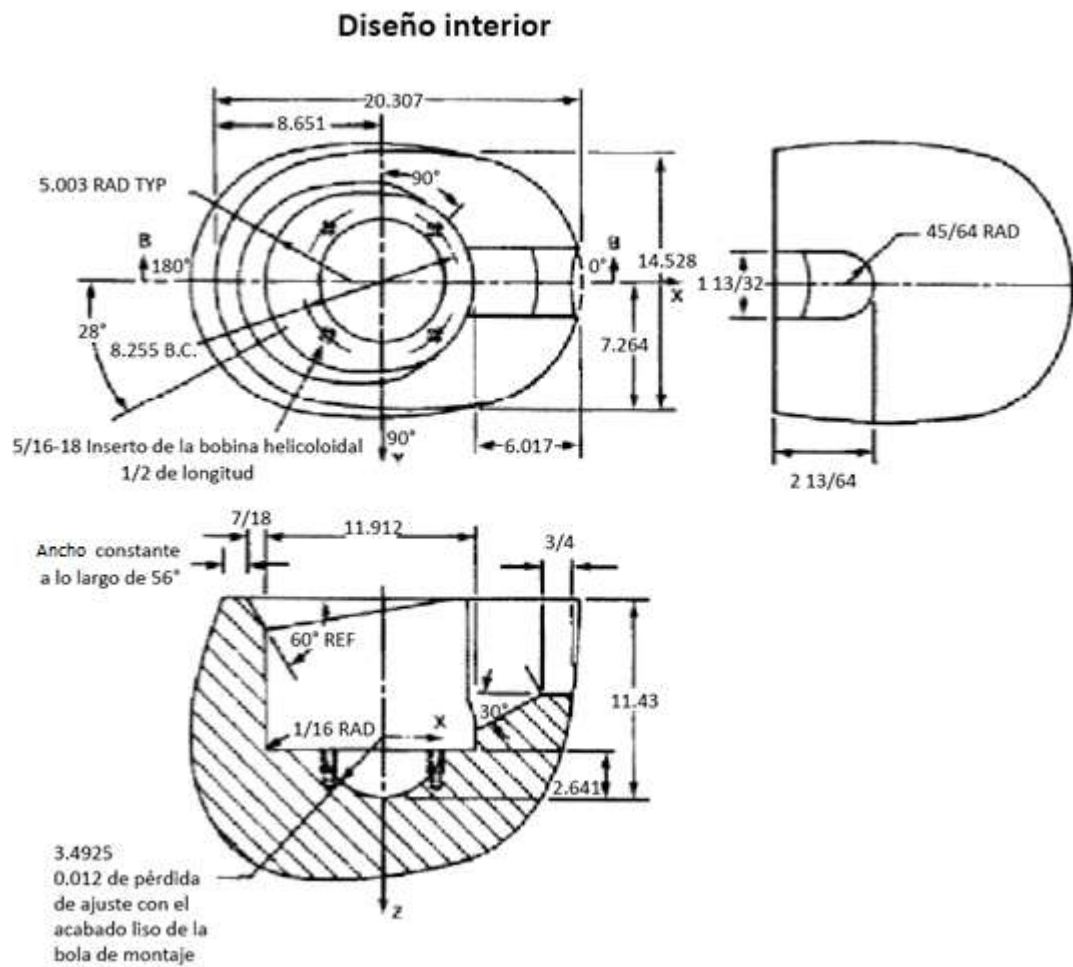
Figura A.5-Cabeza de referencia grande
