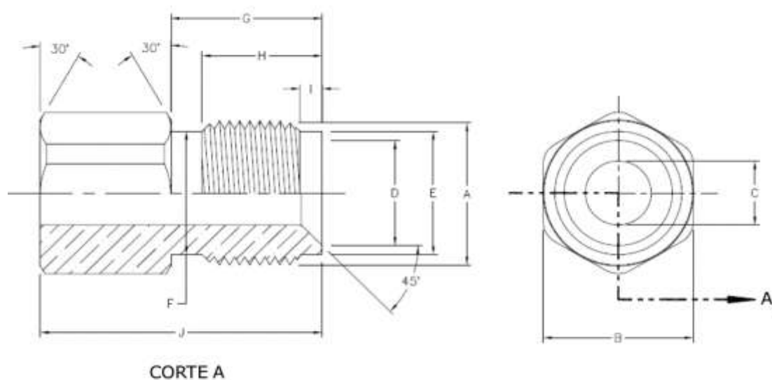
Figura 9-Tuerca con rosca EXT derecha para conexiones Tipo 1 o Tipo 2 (Ilustrativa)
