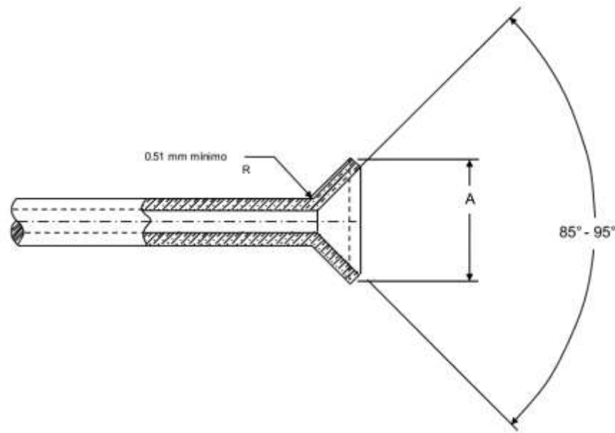
Figura 11-Abocinado del tubo (Ilustrativa)
