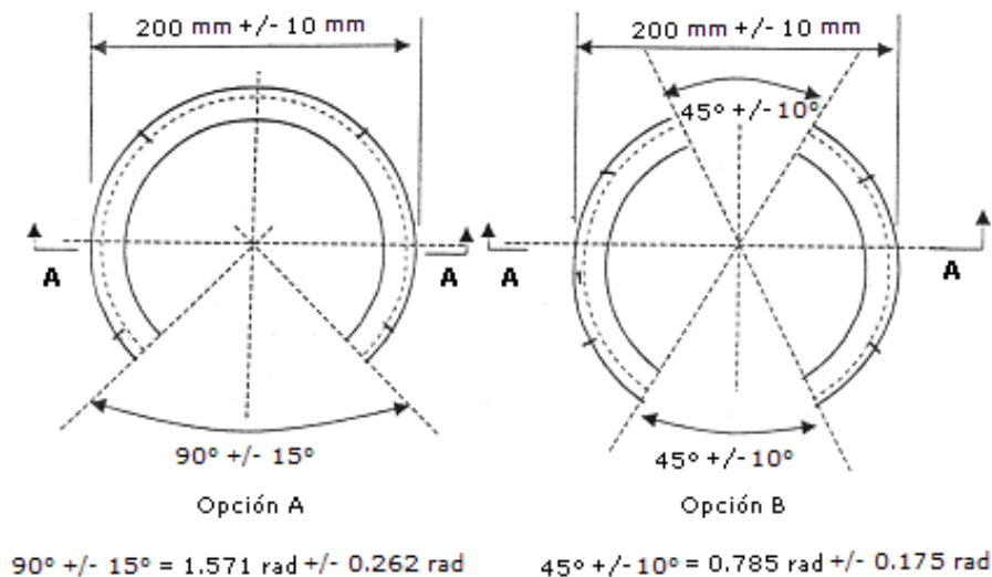
Figura 7- Alternativas de cuello protector para recipiente portátil
