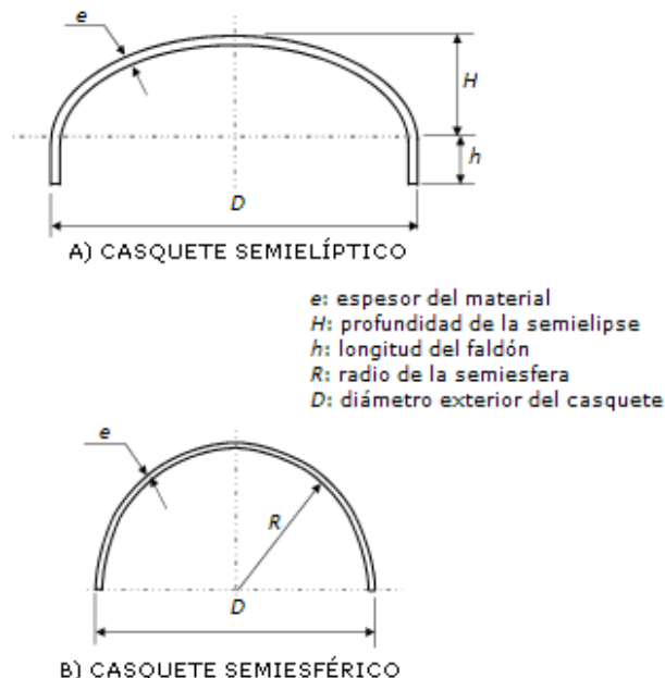
Figura 3- Formas de casquete
