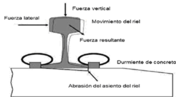
Figura 16-Desgaste de durmiente.
