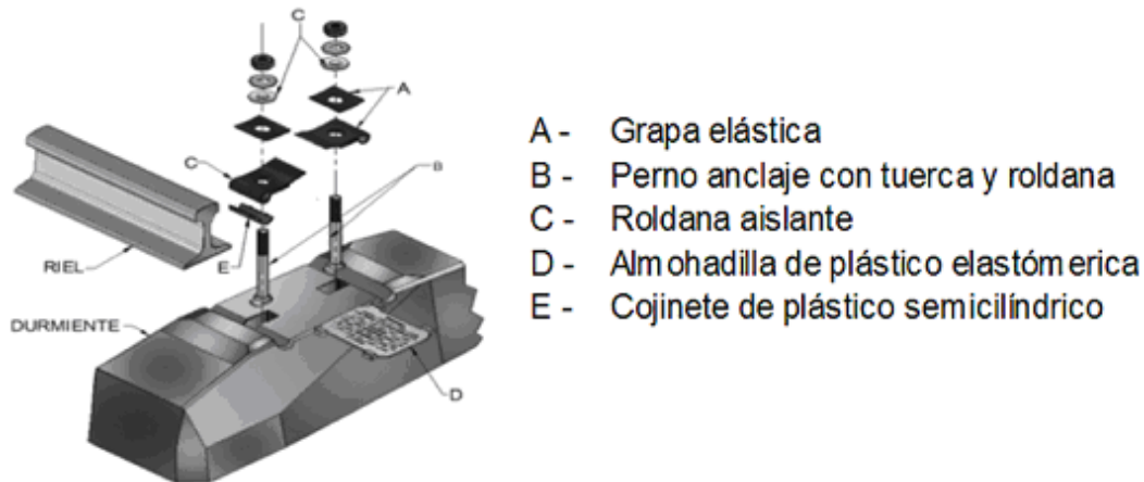
Figura 5-Sistema de fijación en vía elástica
