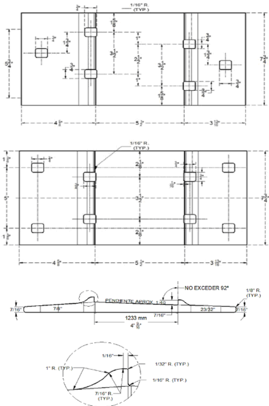
Figura 6-Placas de asiento
