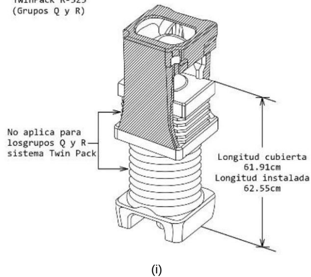
Fig. 4. Áreas críticas para el cilindro exterior.
