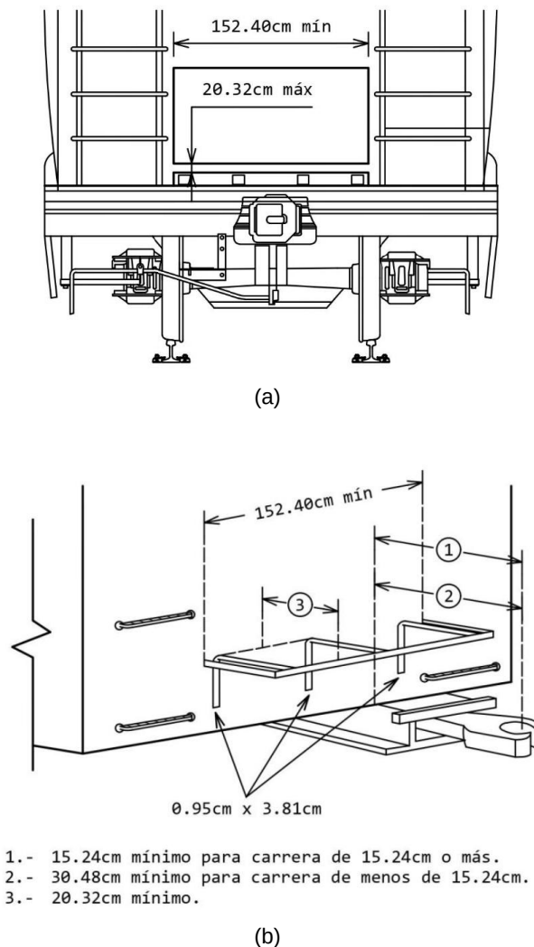
Fig. 15 Repisas transversales de extremo.
