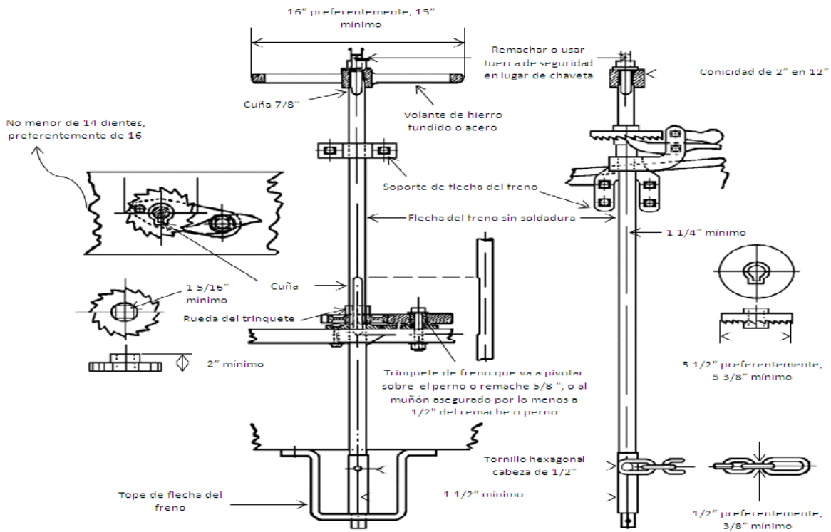
MECANISMO DEL FRENO DE MANO
