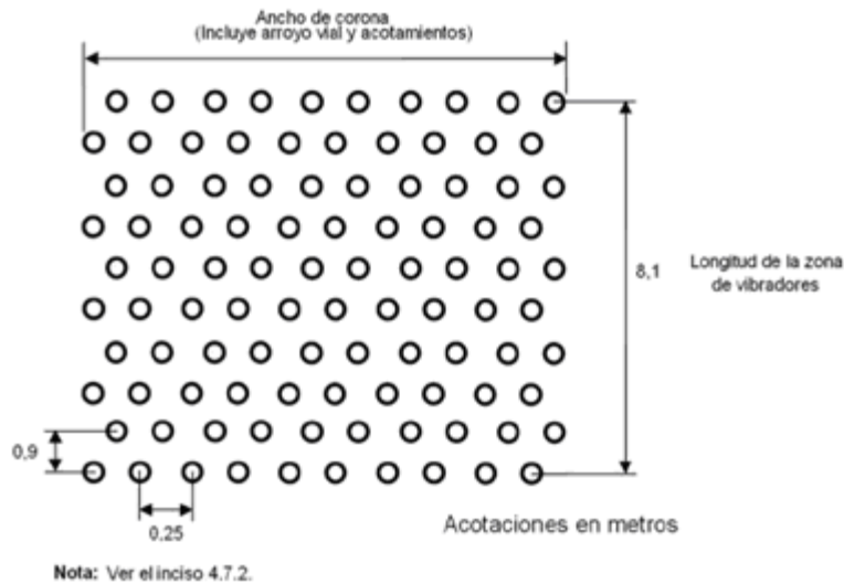
FIGURA 13.- Distribución de los botones (DH-3) en la zona de vibradores
