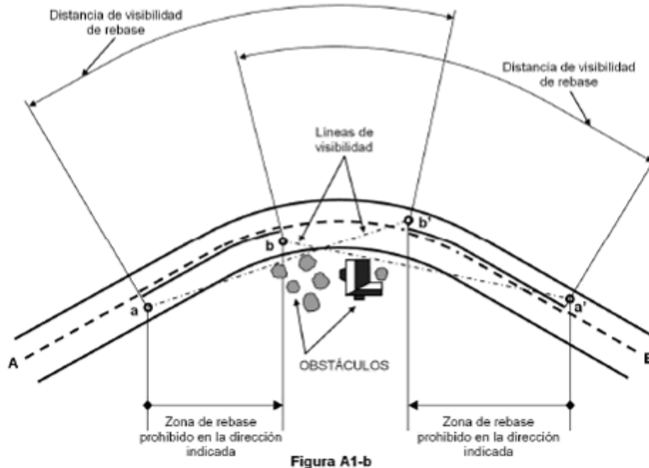
FIGURA A1.- Procedimiento para ubicar los límites de los tramos de rebase prohibido en curvas horizontales
