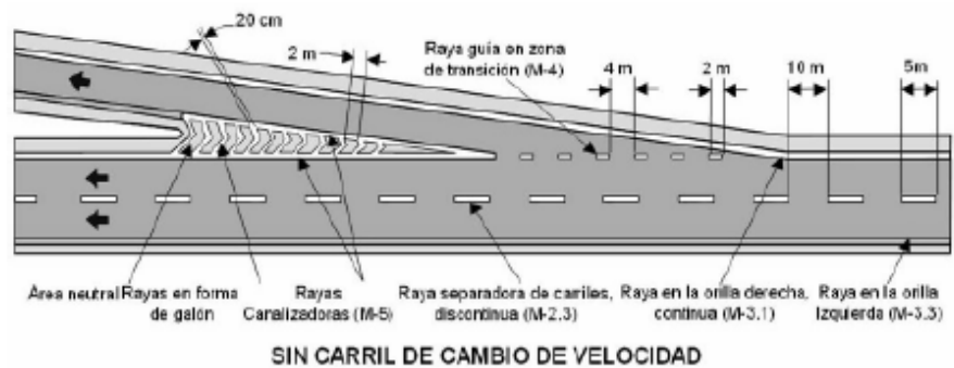
FIGURA 7.- Rayas separadoras de carriles, rayas guía en zonas de transición, rayas canalizadoras y rayas en la orilla del arroyo vial
