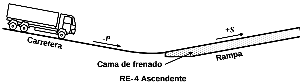
Figura 2.- Tipos de rampas de emergencia para frenado (RE)
