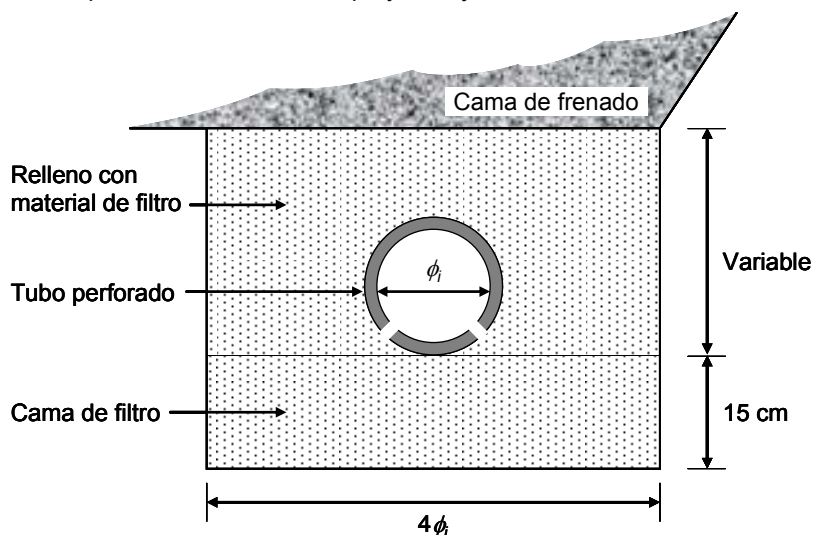
Figura 5.- Subdrén típico para la cama de frenado
