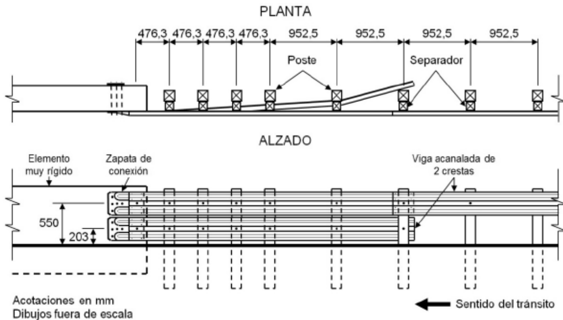
FIGURA 21.- Transición de barrera metálica de doble banda a muro vertical recto
