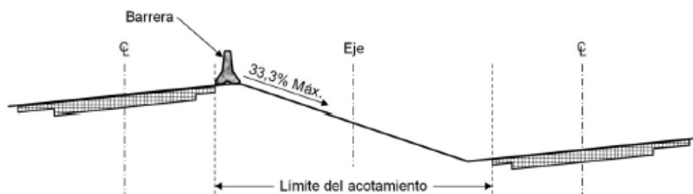
FIGURA 14.- Emplazamiento lateral de barreras separadoras de sentidos de circulación (OD-4.2) en fajas o camellones con pendientes transversales entre 33,3 % y 10% por ciento, sin obstáculos
