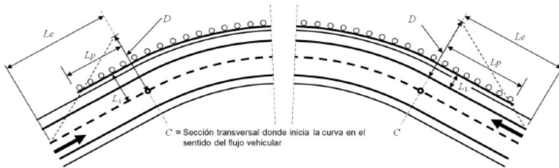
FIGURA 9.- Longitud previa mínima necesaria de barreras de orilla de corona (OD-4.1) para curvas horizontales, circulares o espirales ( L_p )
