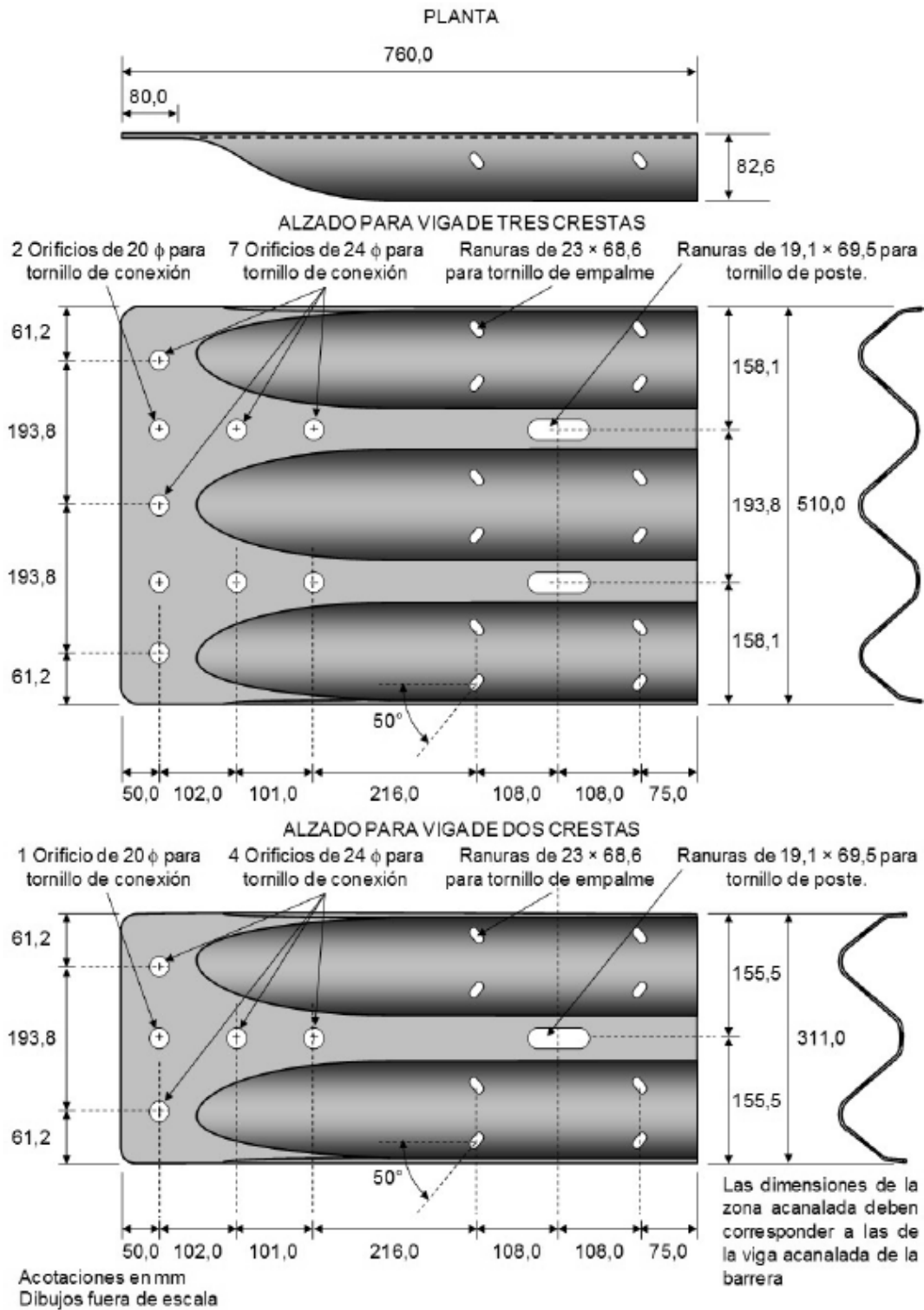
FIGURA 17.- Zapatas de conexión para barreras de vigas acanaladas de acero
