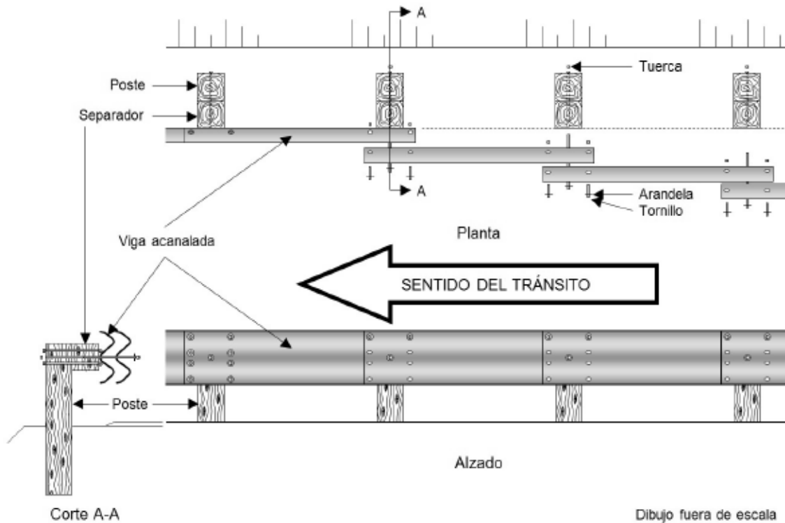
FIGURA 16.- Instalación de vigas acanaladas de acero
