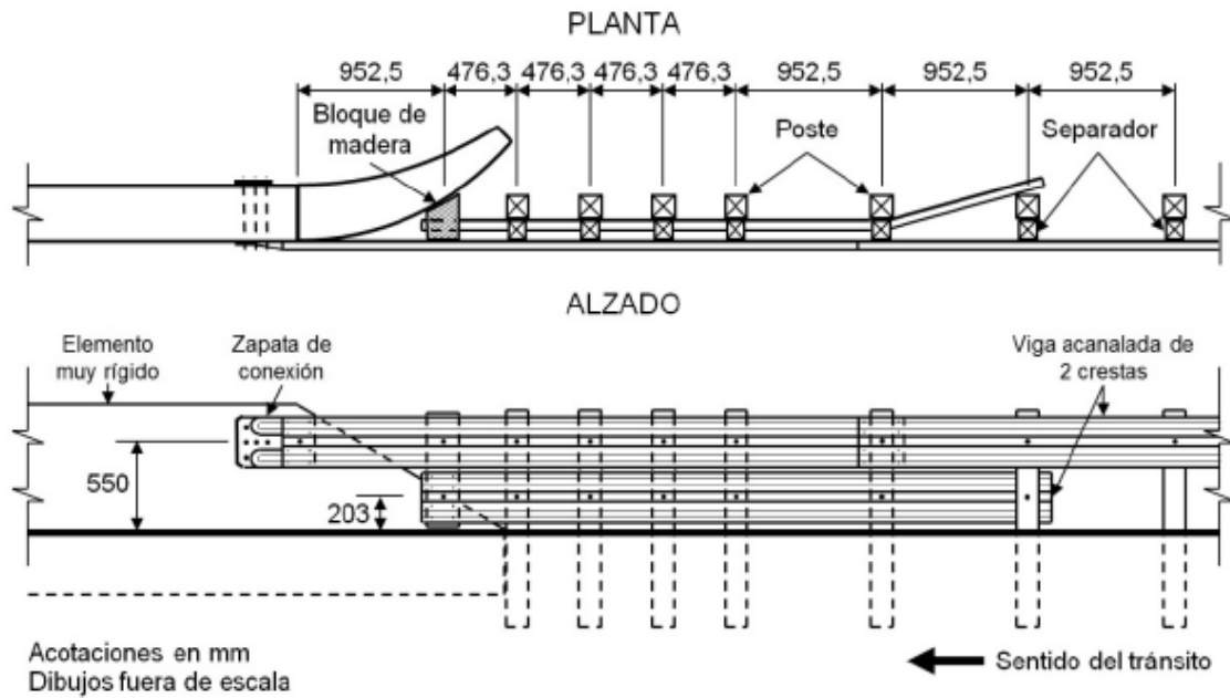
FIGURA 22.- Transición de barrera metálica de doble bandas a muro curvo
