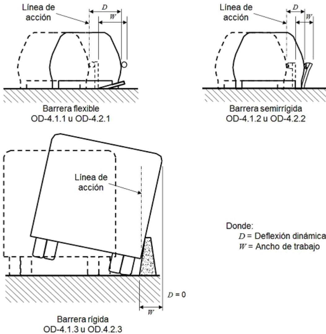
FIGURA 1.- Deflexión dinámica de diferentes tipos de barreras de protección (OD-4)
