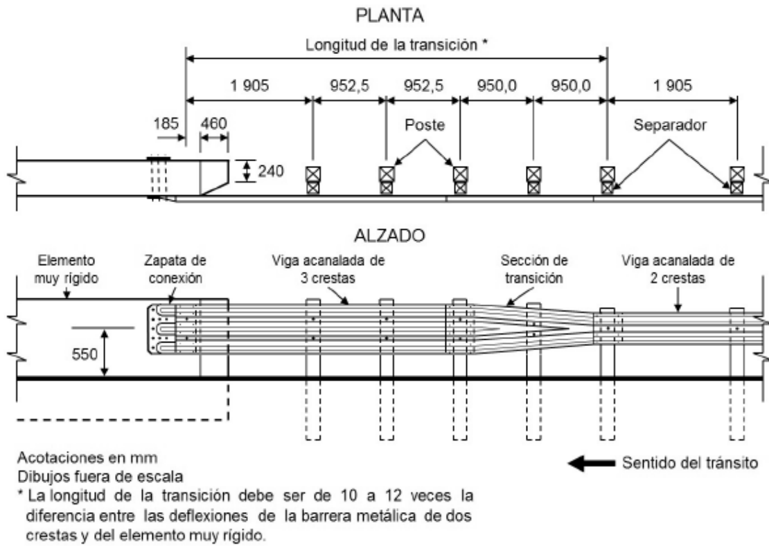
FIGURA 20.- Transición de barrera metálica de dos a tres crestas y a muro vertical recto
