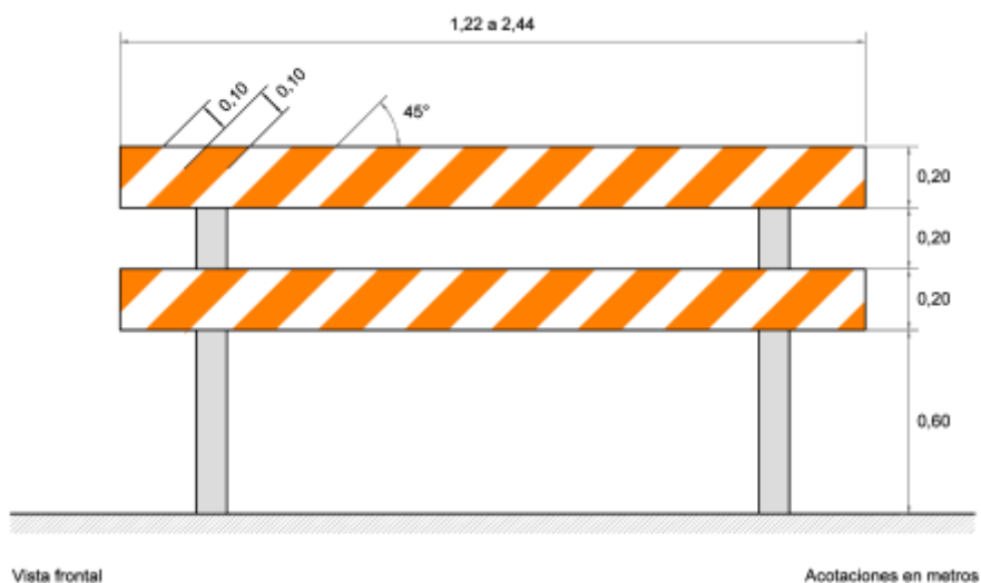
FIGURA 4.- Barrera fija
