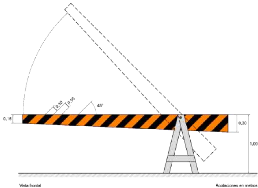
FIGURA 3.- Barrera levadiza
