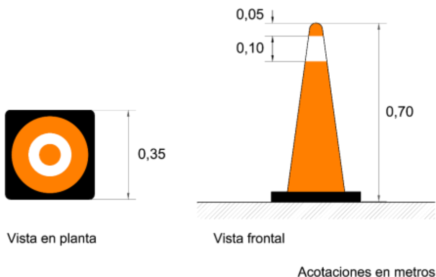
FIGURA 7.- Cono
