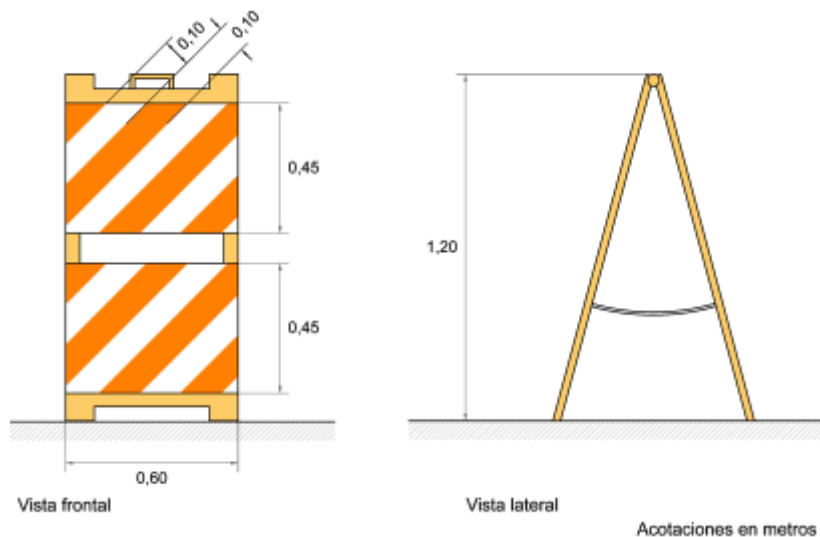
FIGURA 5.- Caballete
