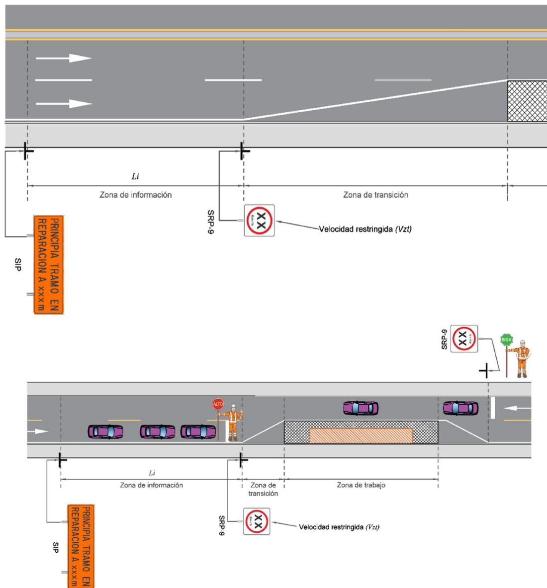
FIGURA 23.- Señales verticales que indican el principio y fin de la zona de información (Li)
