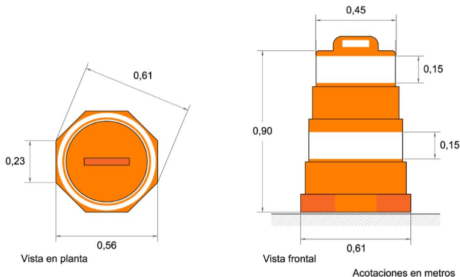
FIGURA 8.- Tambo
