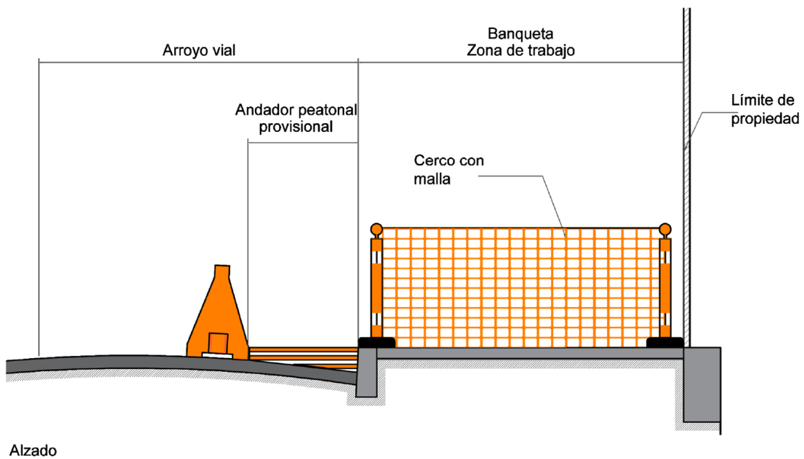
FIGURA 14.- Malla
