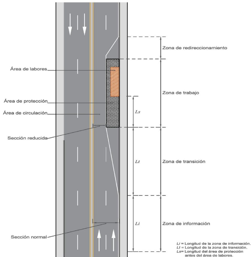
FIGURA 1.- Zona de obra en carreteras
