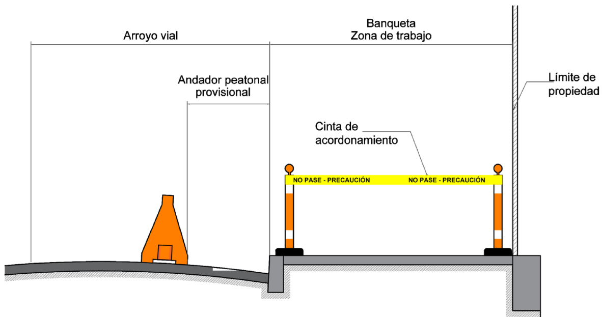
FIGURA 15.- Cinta de acordonamiento
