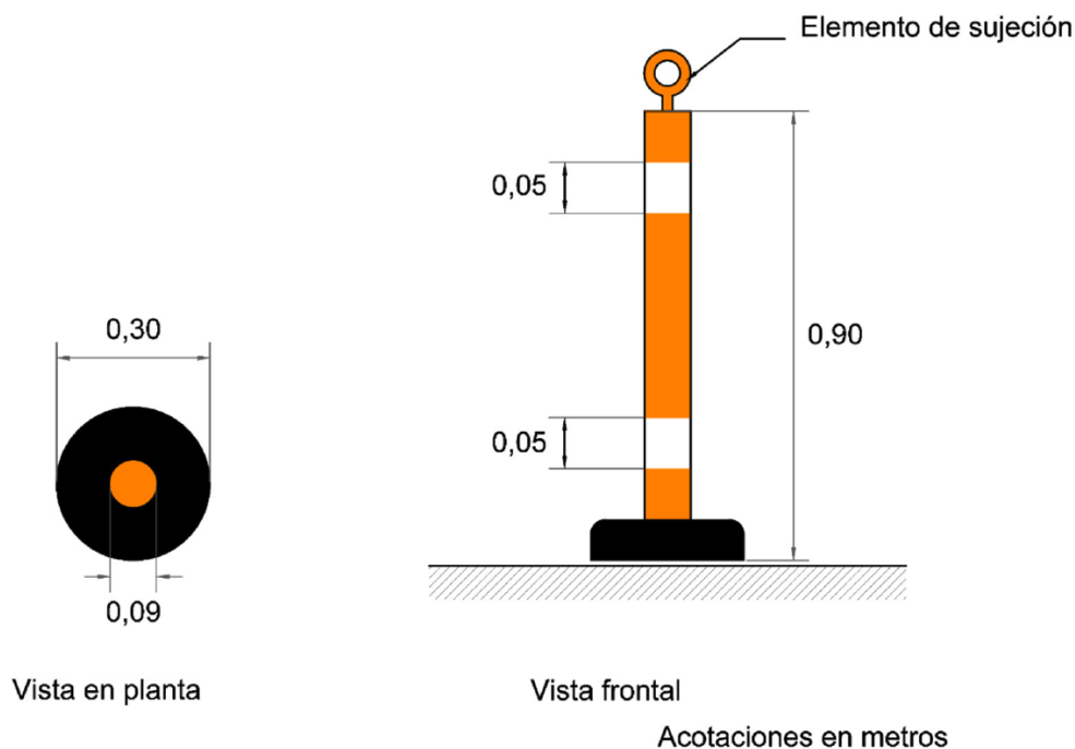
FIGURA 18.- Baliza delineadora
