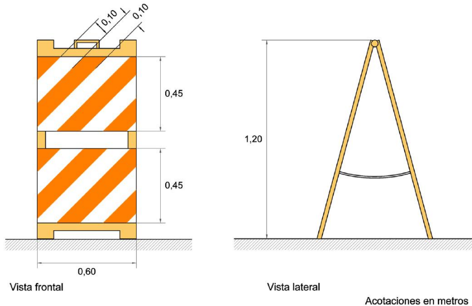
FIGURA 5.- Caballete
