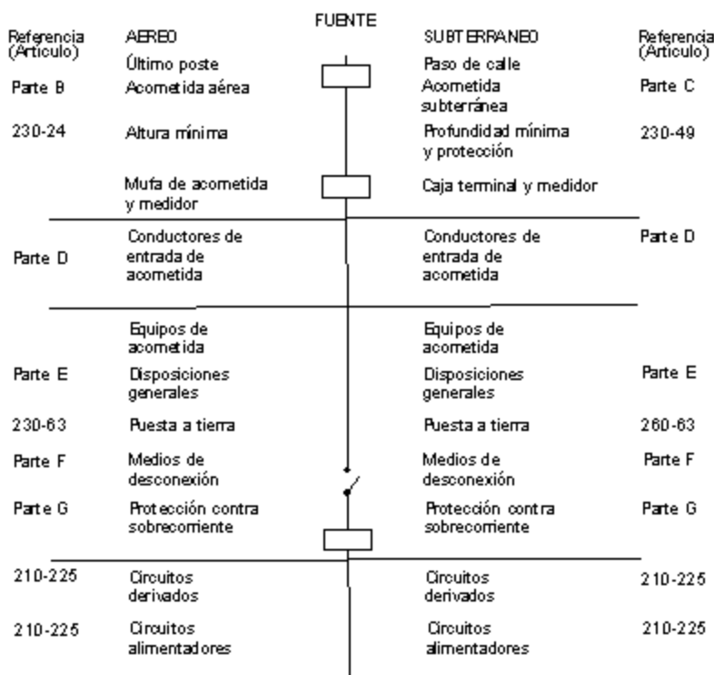
FIGURA 230-1.- Acometidas
