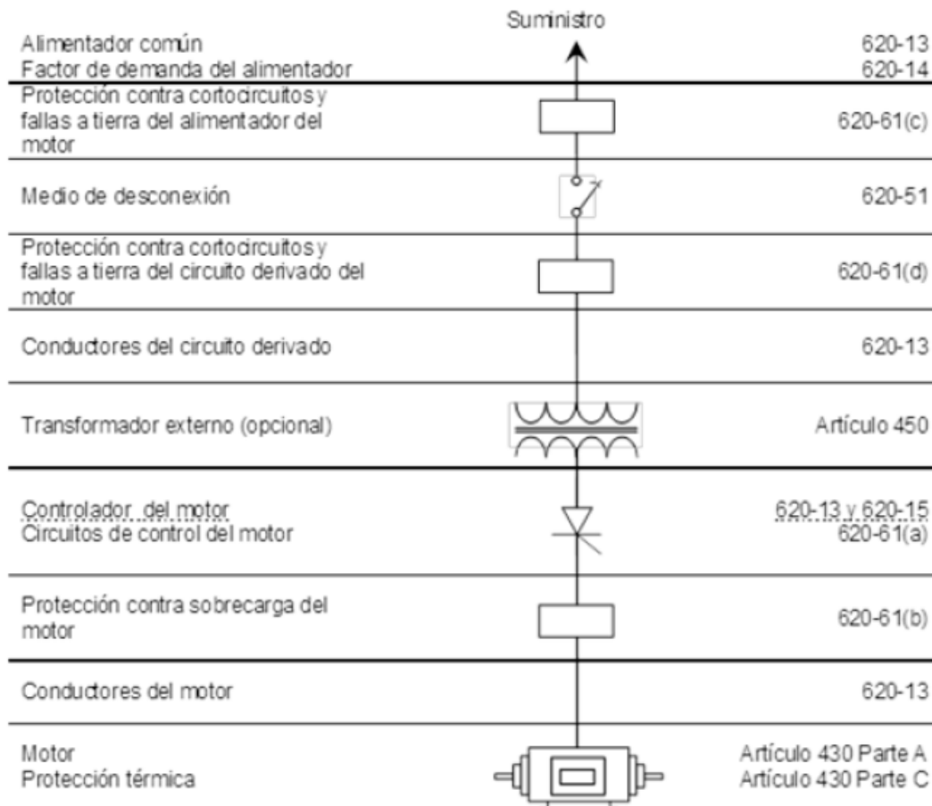
Figura 620-13.- Diagrama unifilar
