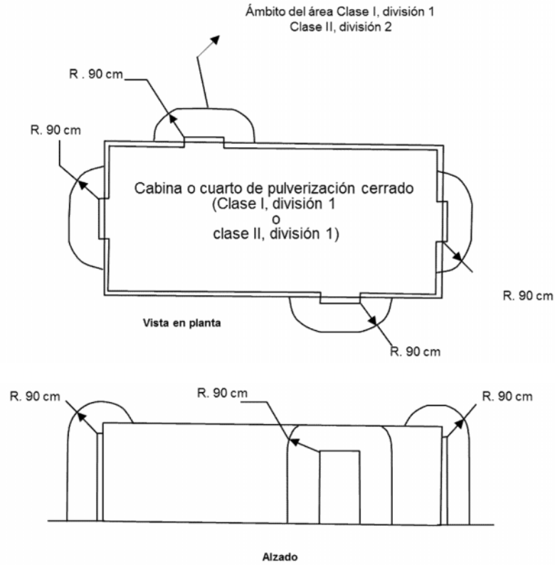
Figura 516-3(c)(2).- Areas Clase I, División 2; Clase I, Zona 2 o Clase II, División 2 adyacentes a un recinto o una cabina del rociado cerrados por arriba, abiertos por la cara o abiertos por el frente
