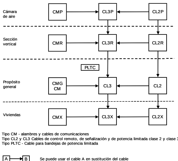
FIGURA 725-61.- Jerarquía de sustitución de los cables
