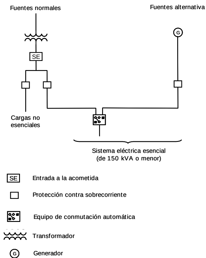
FIGURA 517-41(b).- Sistema eléctrico grande en lugares para enfermería y áreas de atención limitada
