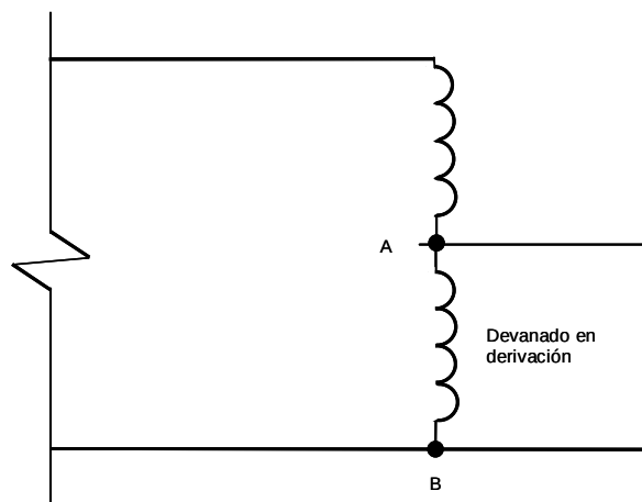
FIGURA 450-4.- Autotransformador
