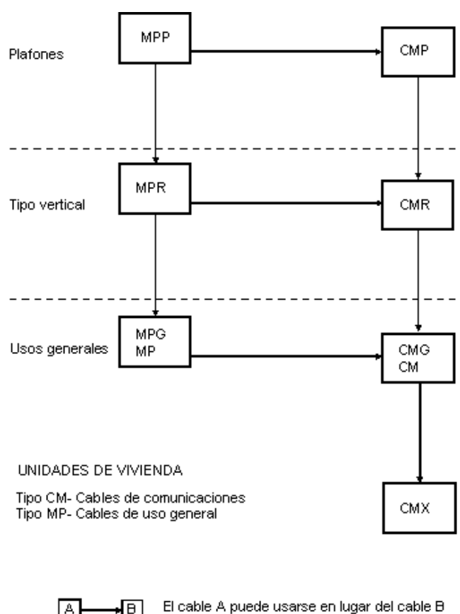
Figura 800-53.- Jerarquía de sustitución de cables
