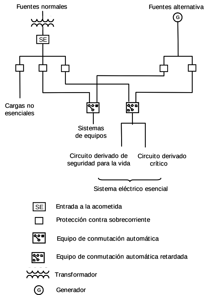
FIGURA 517-30(a).- Sistema eléctrico pequeño - hospitales
