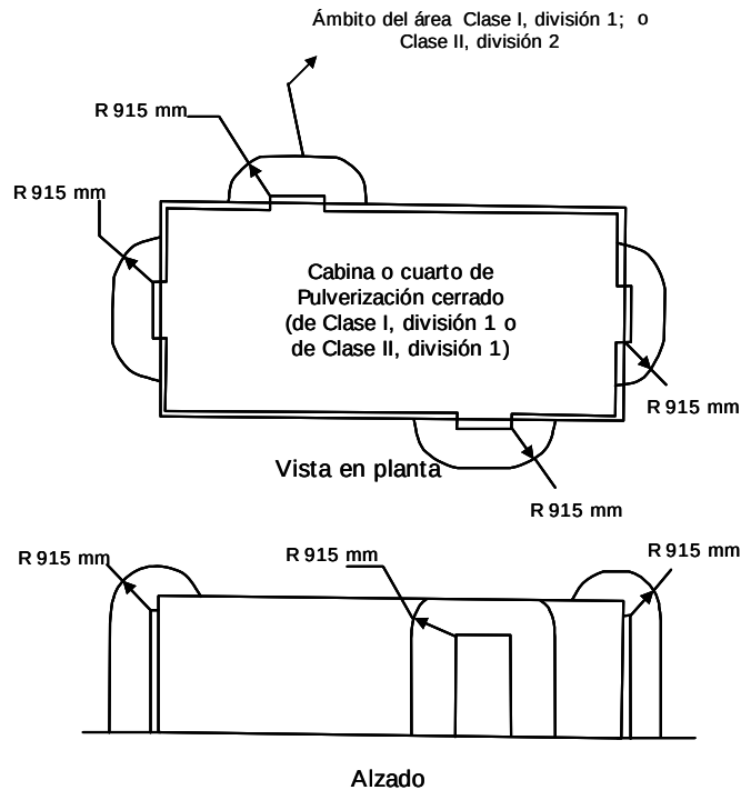
FIGURA 516-2(b)(4).- Areas Clase I (o Clase II) adyacentes a una cabina de rociado cerrada
