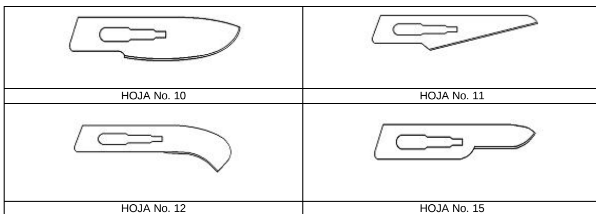
FIGURA 2. HOJAS PARA BISTURÍ (NO IMPLICA DISEÑO) GRUPO 1 (RANURA CHICA)
