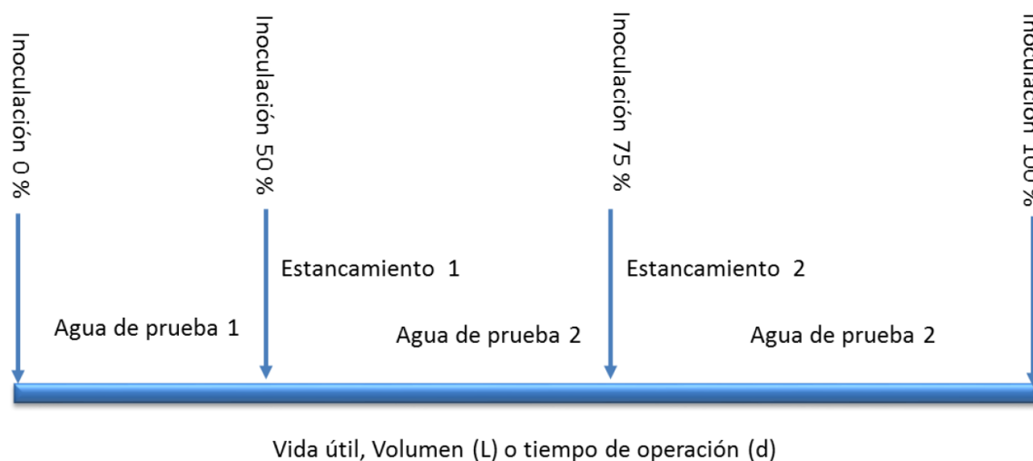
Figura A.3. Verificación en operación continua de la Eficiencia en Reducción Bacteriana en equipos domésticos
