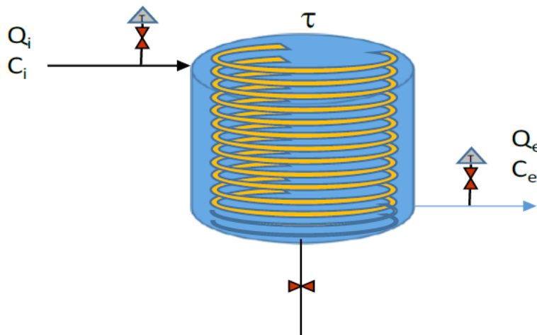
Figura A.4. Variables de operación de un sistema por Lotes.
