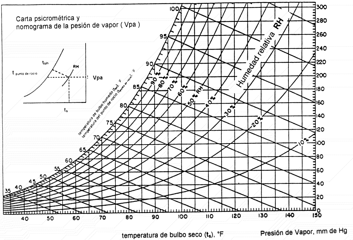
Carta psicrométrica
