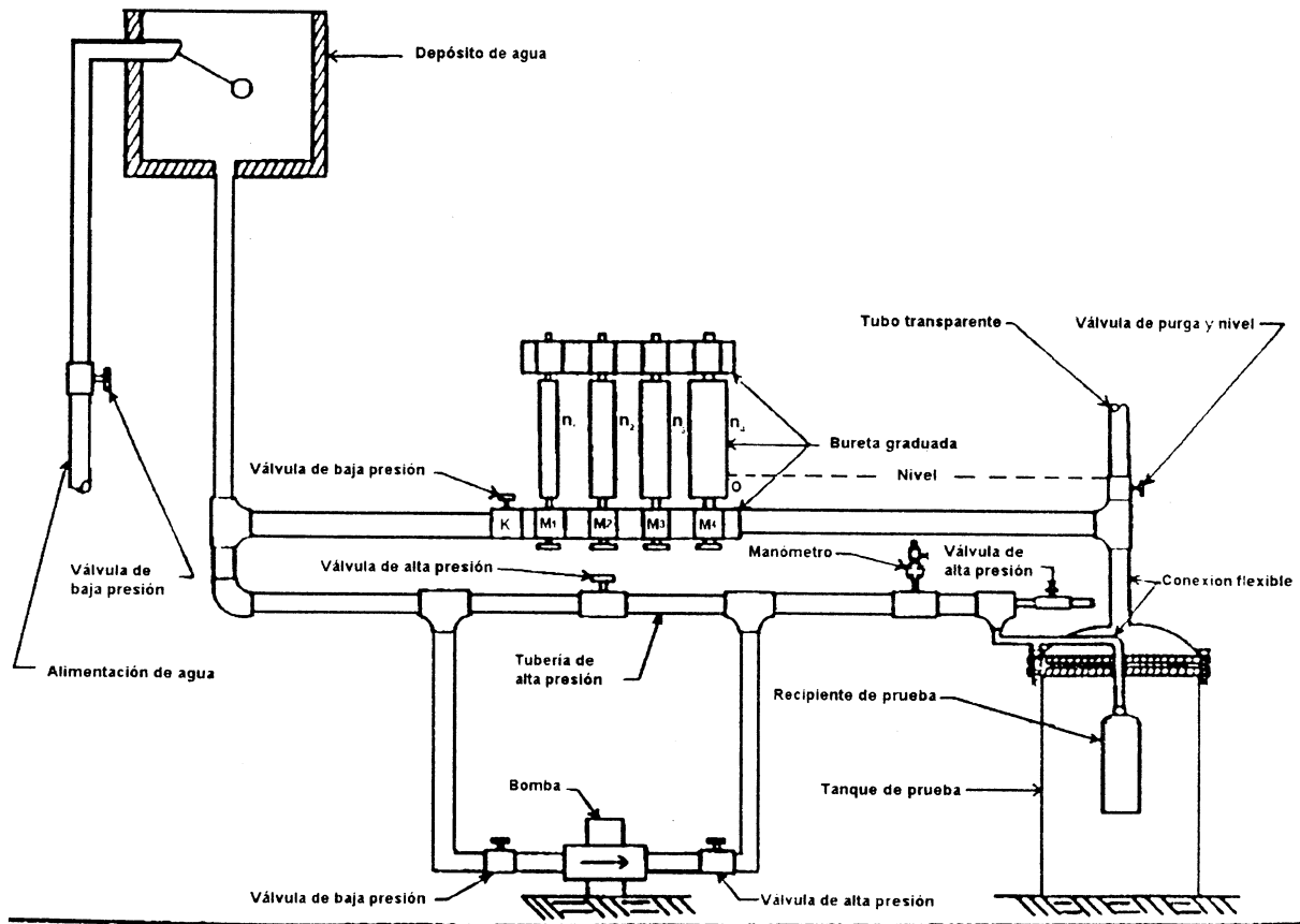
FIGURA 1 PRUEBA DE FORMACIÓN PERMANENTE
