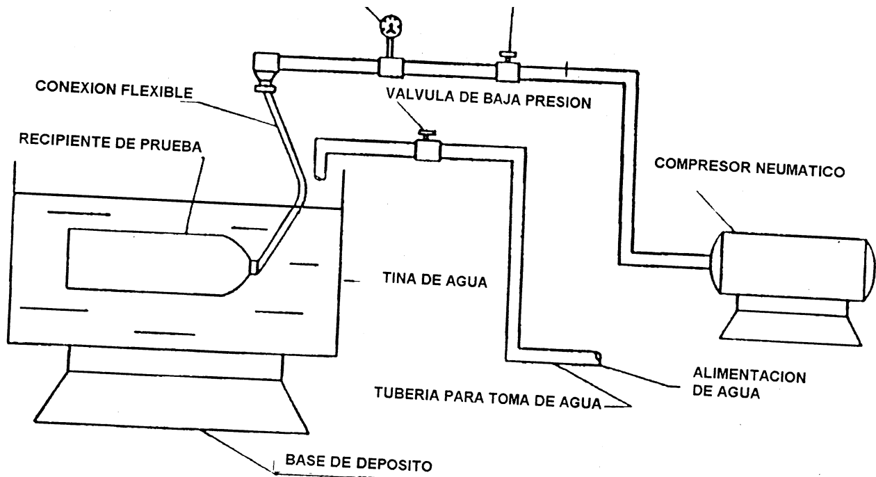
Equipo No. 1 PRUEBA DE HERMETICIDAD
